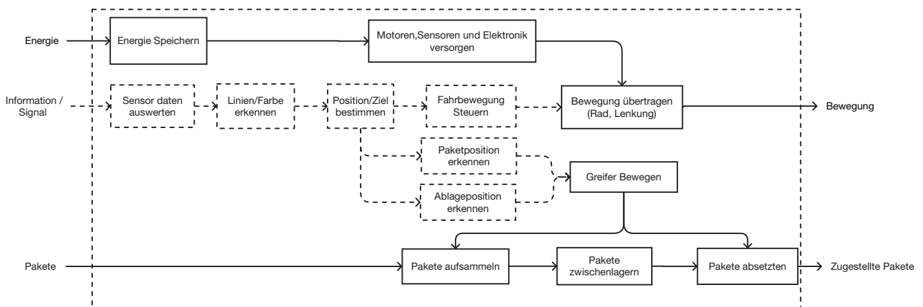
Abbildung 2: Funktionsstruktur
