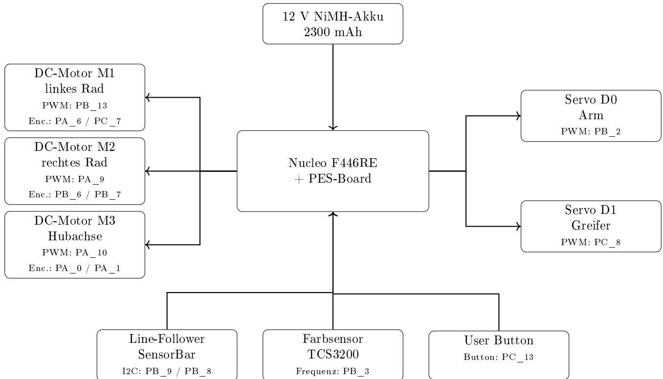
Abbildung 6: Vereinfachtes Elektrodiagramm des Roboters
